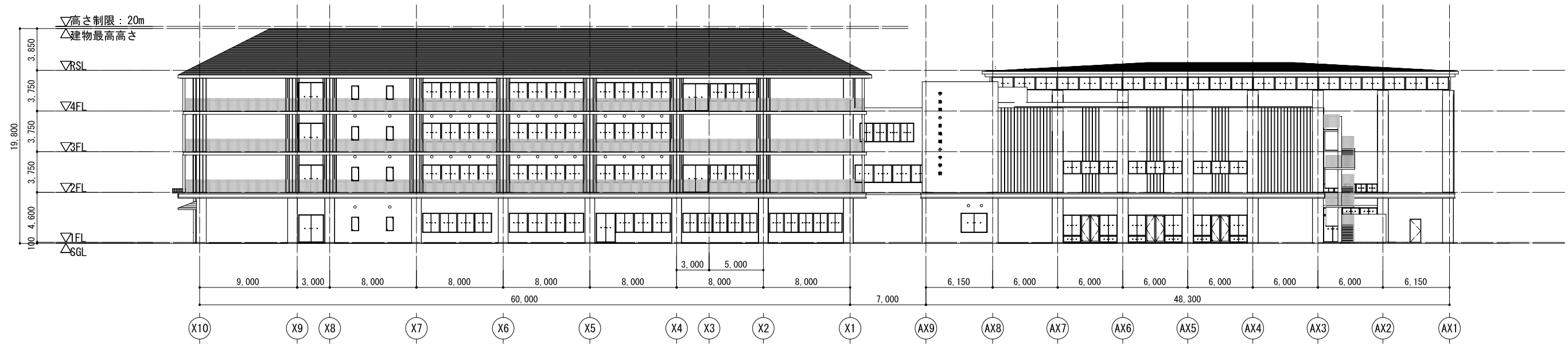
A-A' 北立面図
