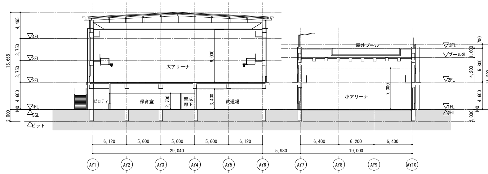
D-D断面図
