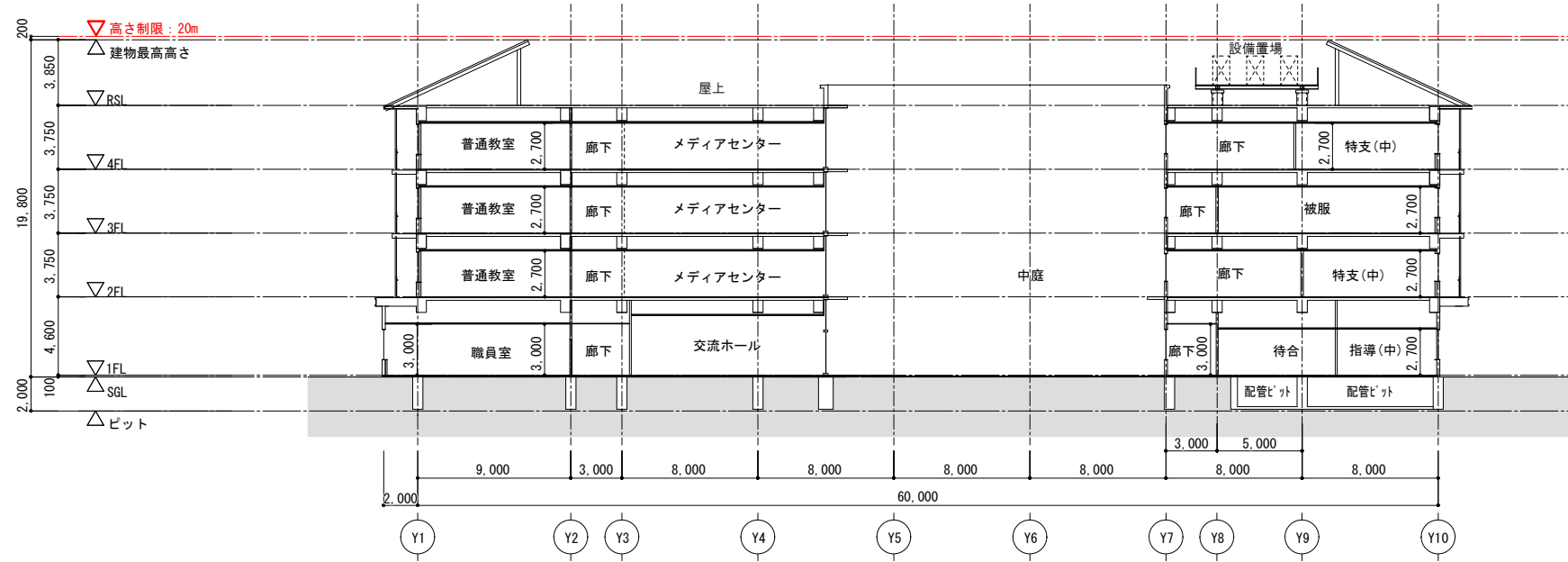
C-C断面図
