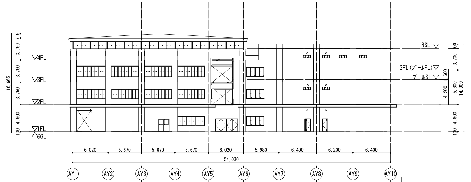
E-E' アリーナ棟 東立面図
