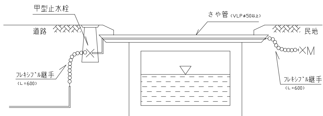
図 5－7 水路上越し配管例
