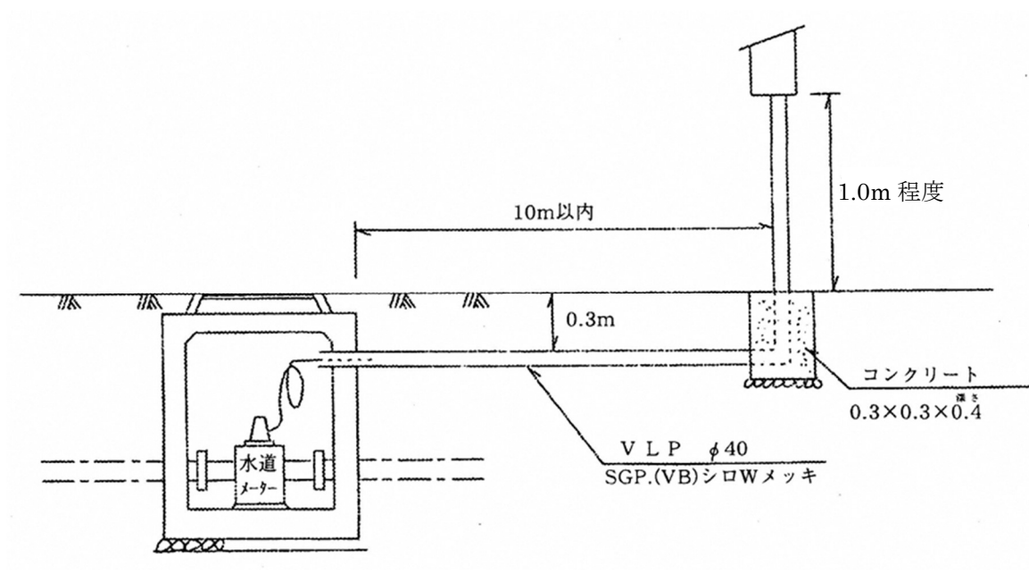
図 5 - 3 遠隔装置盤設置標準図
