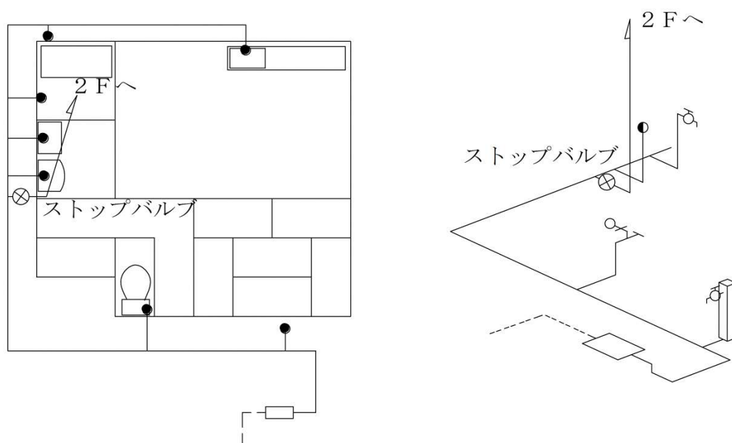
図 5 - 1 0 2 階配管例
