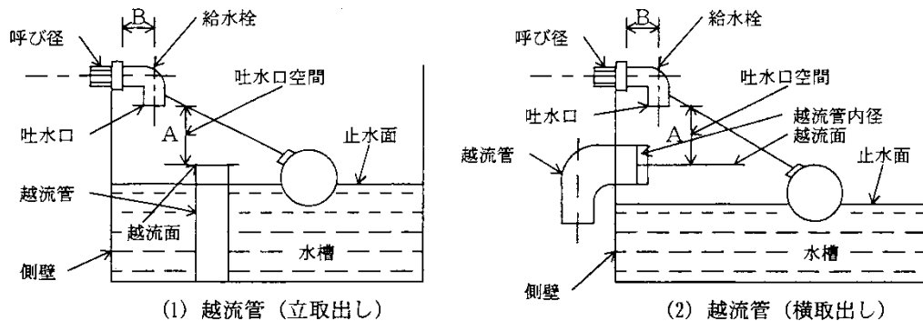
図 7 - 3 水槽の場合
