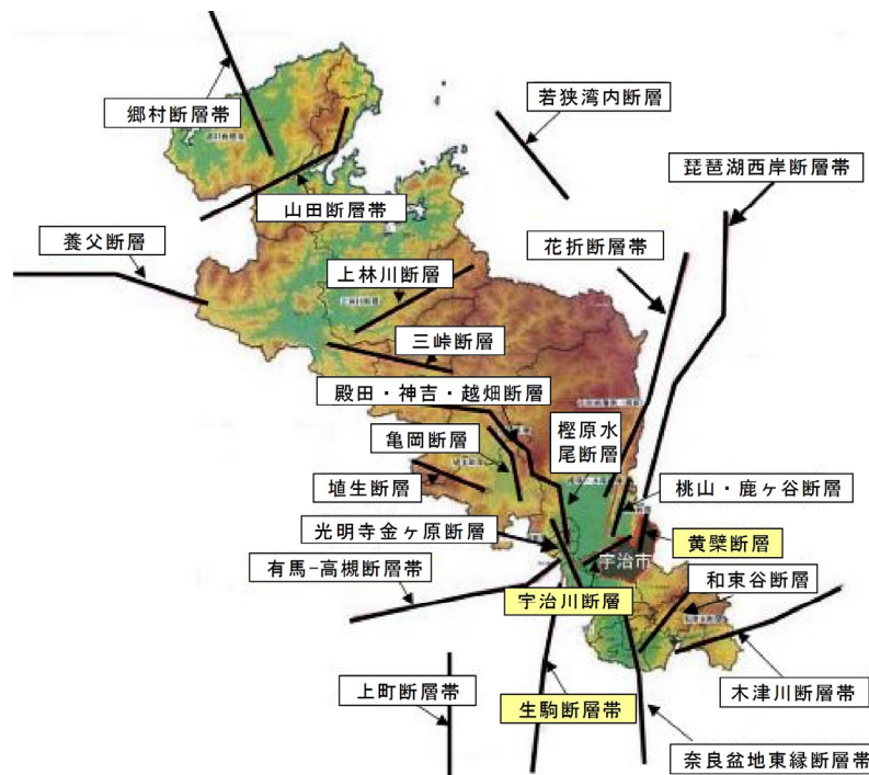
断層分布図
