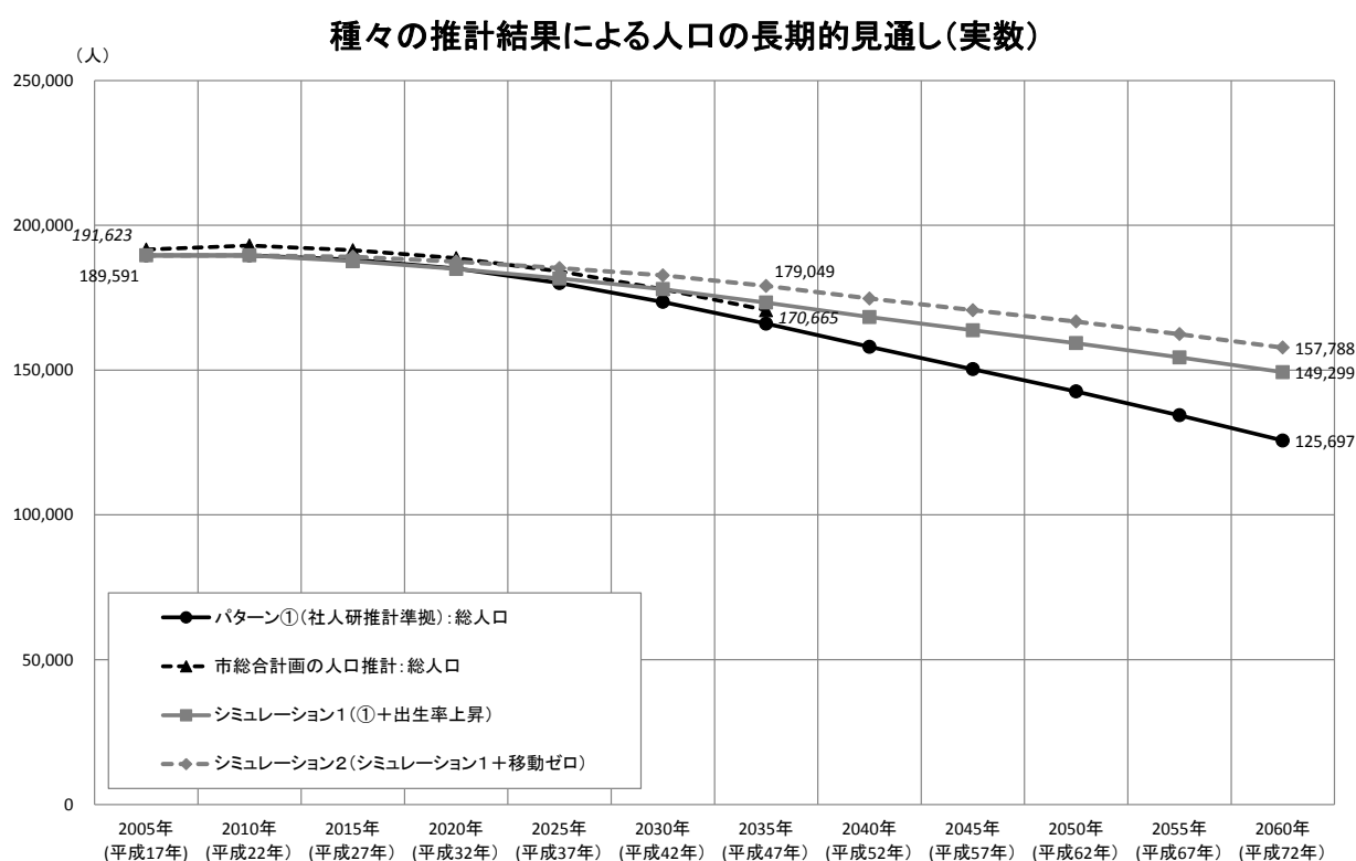
図表 I-18 人口推計結果の比較
