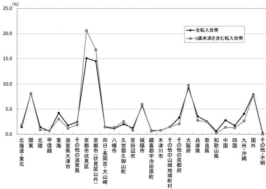
図表 I-15 転出先別に見た転出世帯の割合
