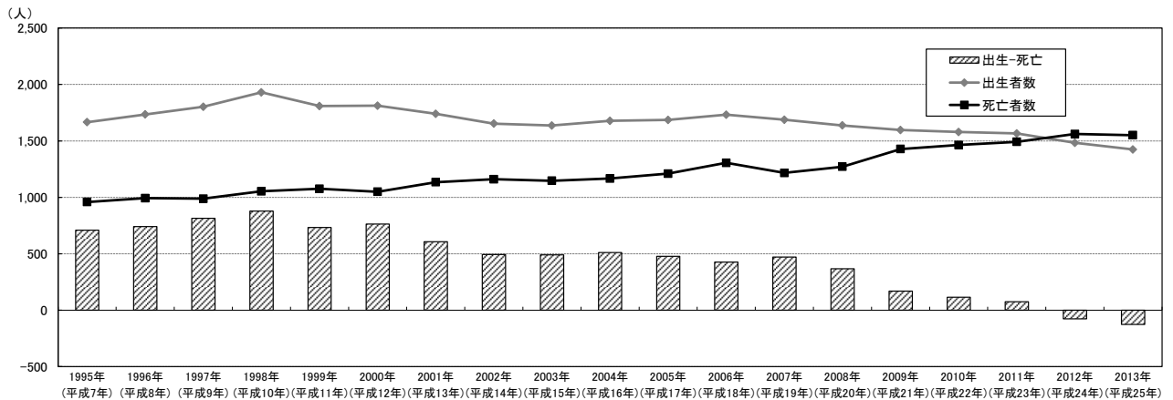
図表 I-6 宇治市における出生・死亡数の推移
