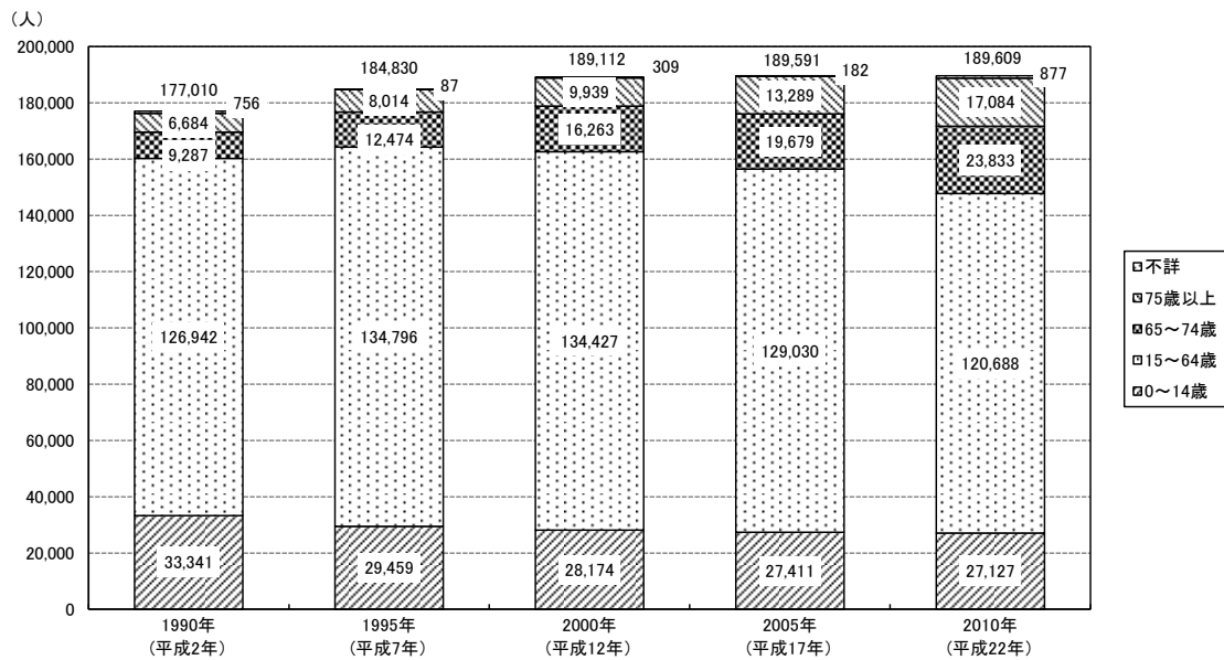
図表 I-3 年齢4区分別人口
