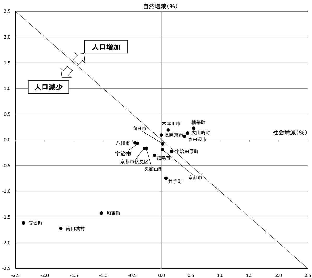
図表 I-5 京都府南部における人口増減の要因（平成25年）
