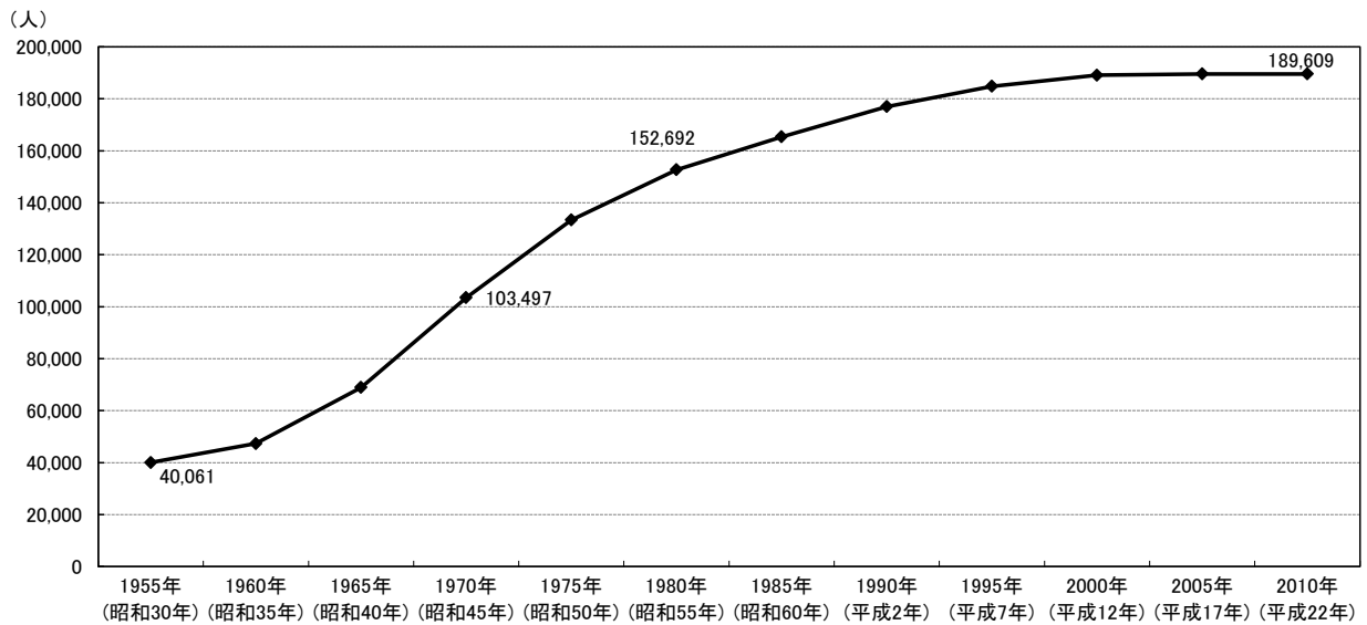
図表 I-1 国勢調査人口
