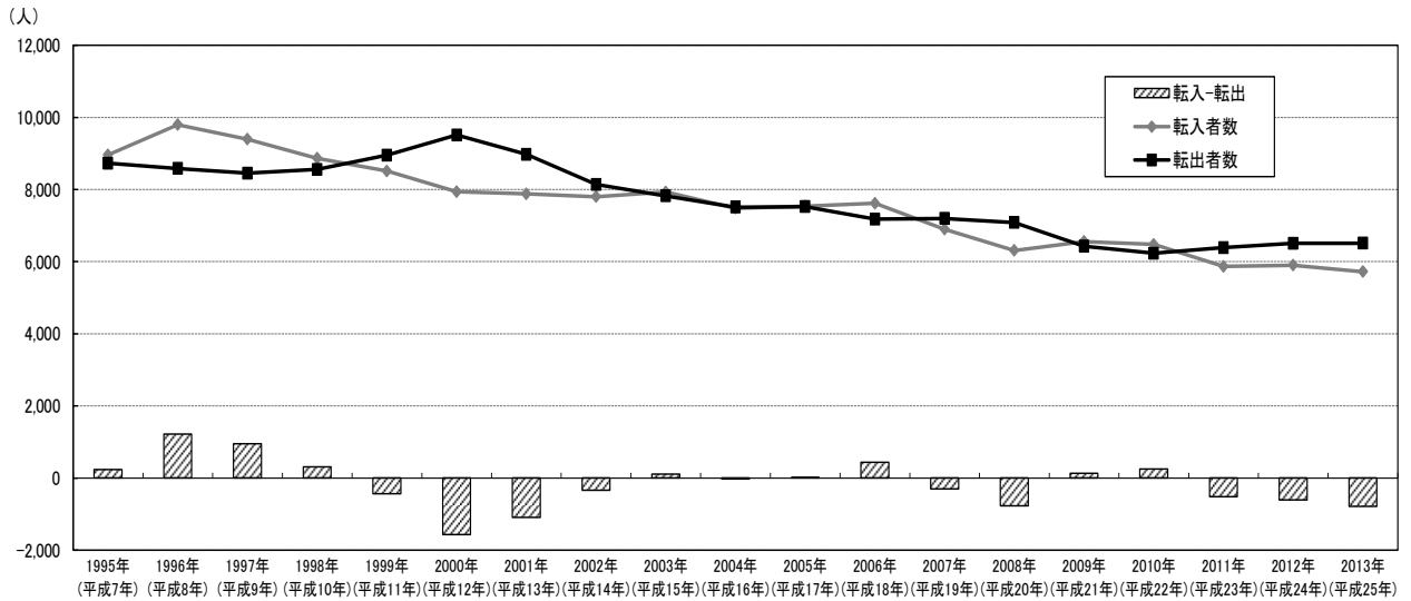
図表 I-10 宇治市に転入・転出数の推移
