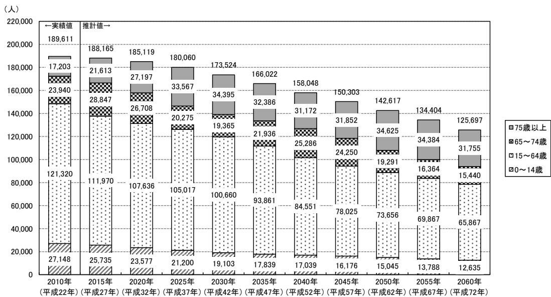
図表 I-16 宇治市における将来推計人口（社人研推計）
