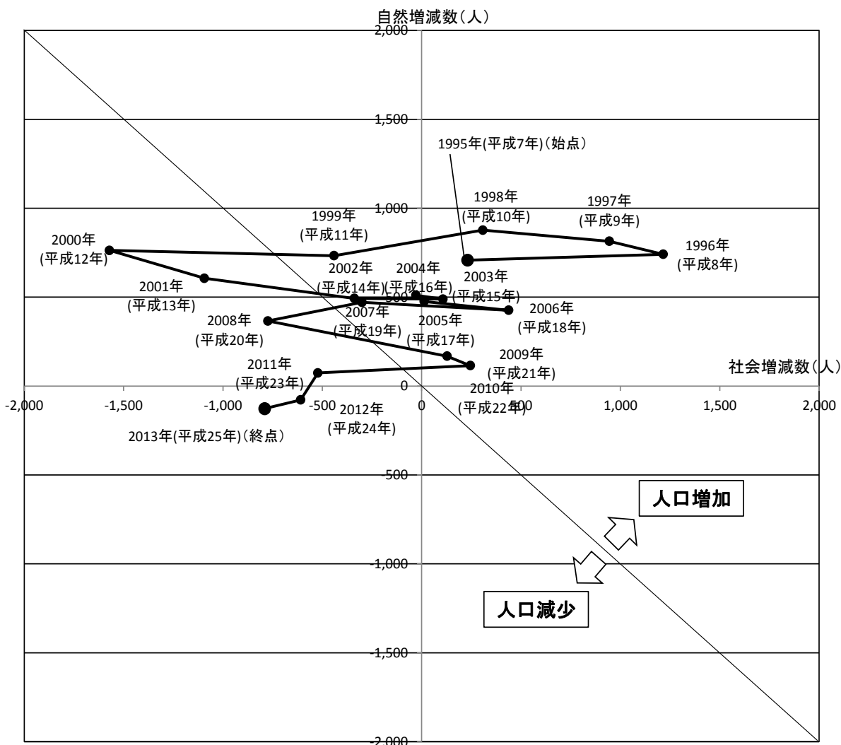
図表 I-4 宇治市における人口増減の要因
