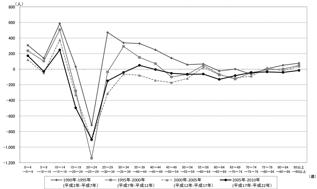
図表 I-13 宇治市における性別・年齢5歳階級別純移動数の推移 男性
