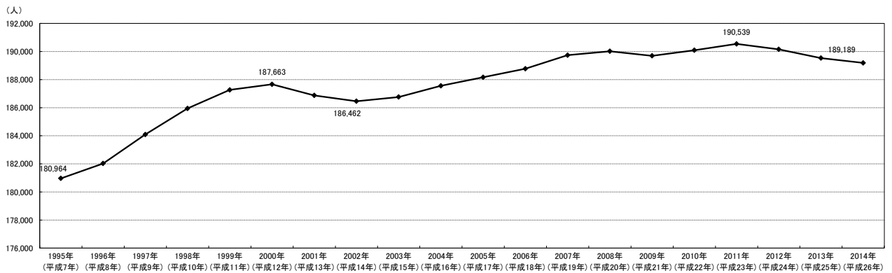
図表 I-2 住民基本台帳人口
